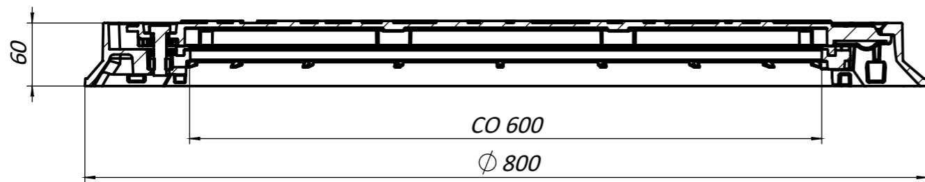
A-A 1:5
